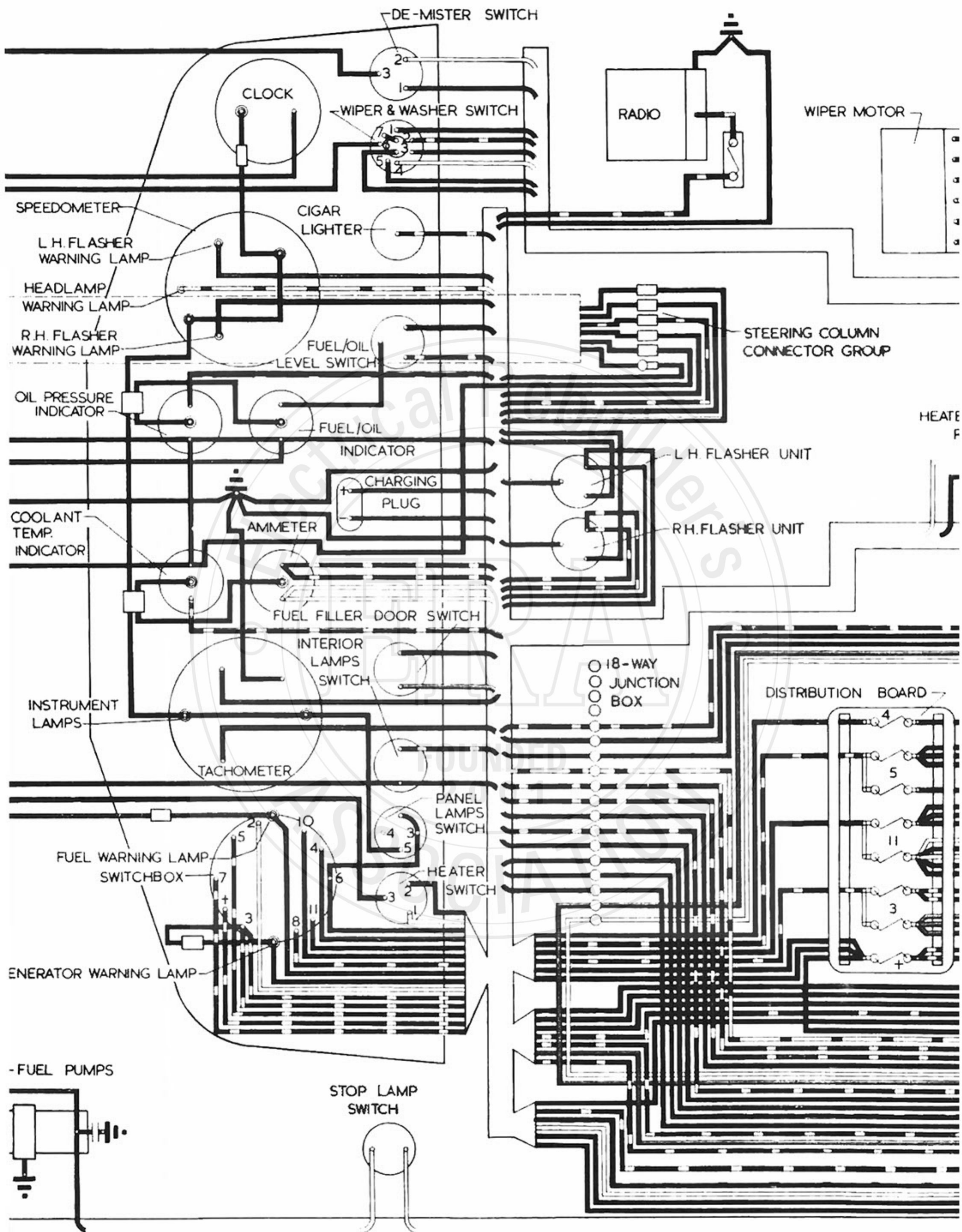
WIRING DIAGRAM—BENTLEY
