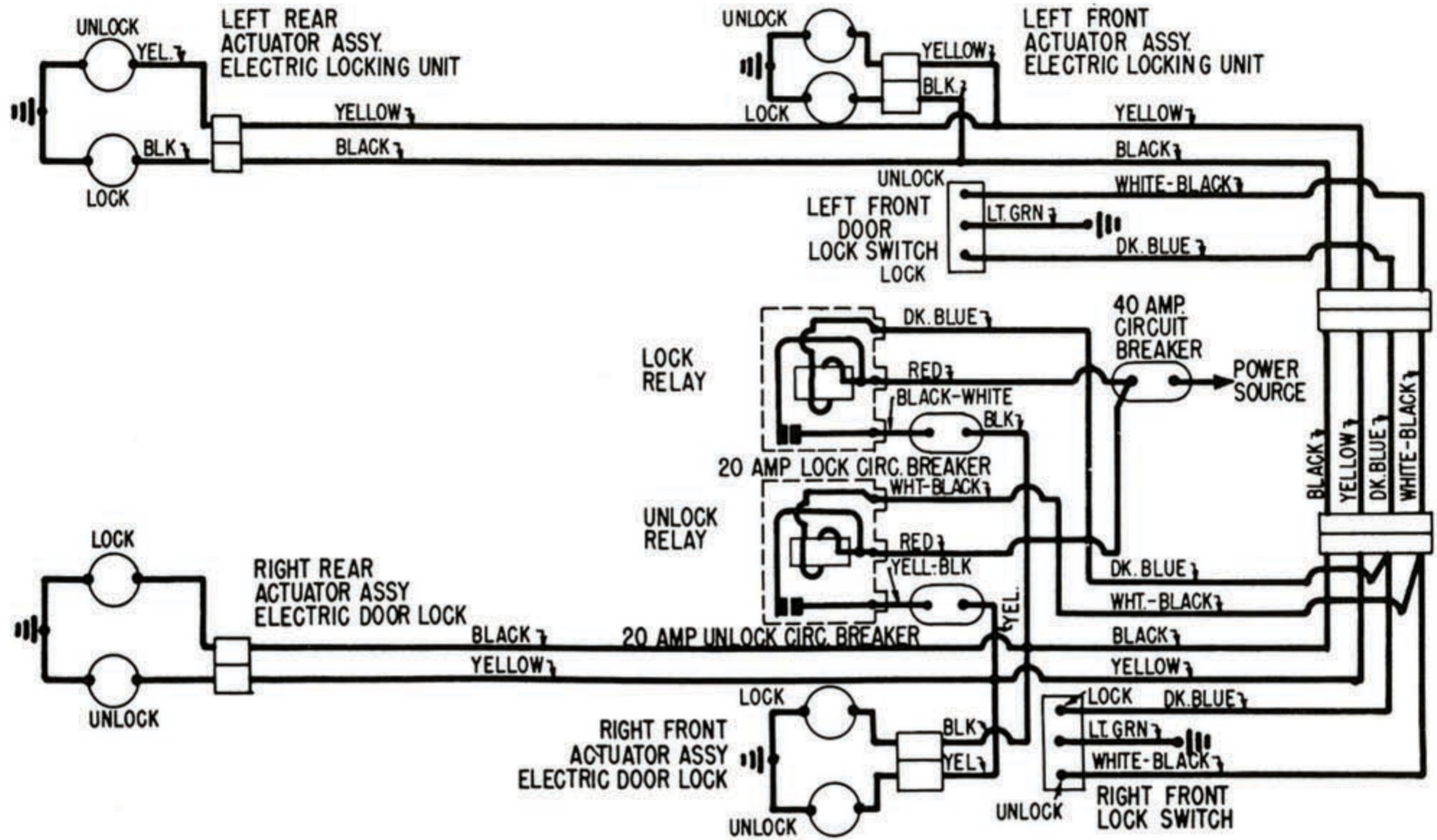
CADILLAC DOOR LOCK WIRING DIAGRAM
