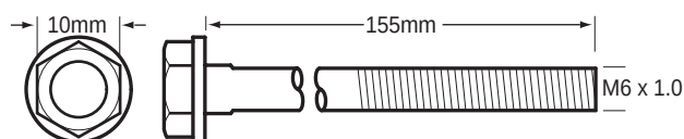
85-1370 Thru Bolt
