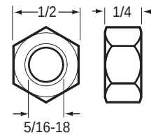
84-2407-1 Hex Nut
