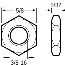
84-2500 Hex Nut
