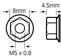
85-2300 Hex Nut
