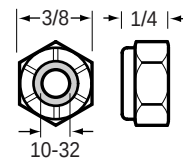
84-2307 Hex Nut
