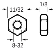
84-2200 Hex Nut
