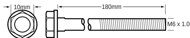
85-1328 Thru Bolt
