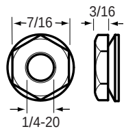
84-2401 Hex Nut
