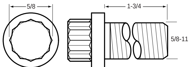
84-1600 Bolt
