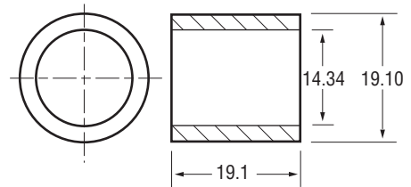
62-1504 Bushing - D.E., C.E.
