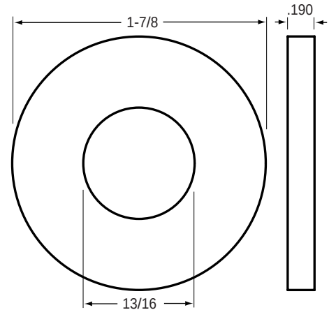
84-7707 Brake Washer
