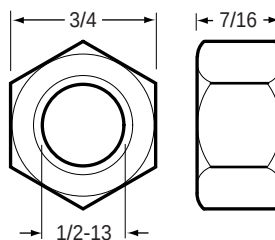
84-2603 Hex Nut
