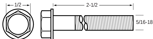
84-1423 Screw
