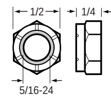
84-2409 Hex Nut
