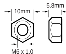
85-2307 Hex Nut
