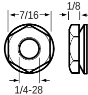
84-2402 Hex Nut
