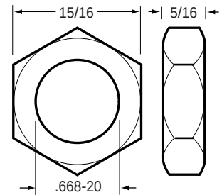
84-2700 Hex Nut
