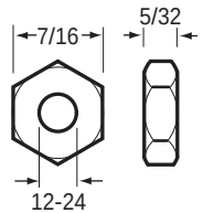
84-2312 Hex Nut
