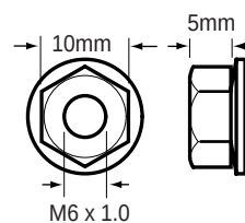
85-2301 Hex Nut
