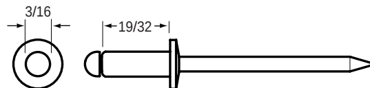
84-3921 Blind Rivet
