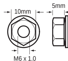
85-2301-2 Hex Nut
