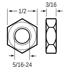
84-2501 Hex Nut
