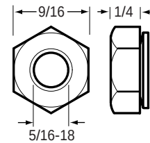
84-2403 Hex Nut
