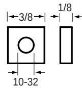
84-2301 Square Nut
