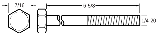
84-1416 Thru Bolt
