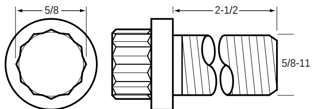
84-1601 Bolt
