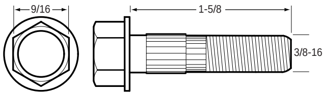
84-1506 Bolt
