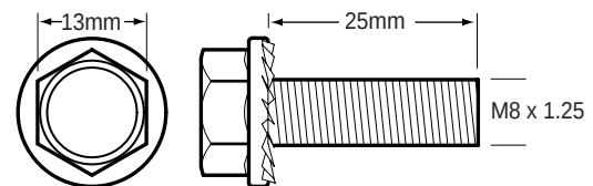
85-1401 Bolt
