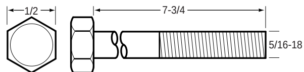
84-1424 Thru Bolt
