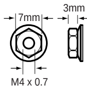
85-2201 Hex Nut
