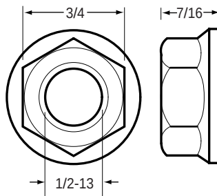
84-2600-1 Hex Nut
