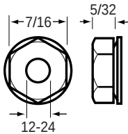
84-2306 Hex Nut
