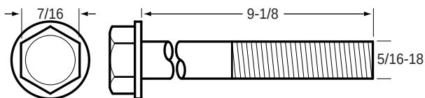
84-1426 Thru Bolt
